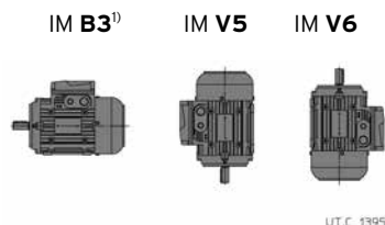
Forme costruttive con piedi - Mounting positions with feet
