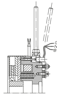
Segnalazione usura freno Brake wear signal
