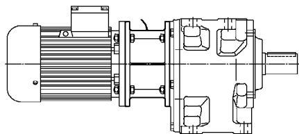
MLA montaggio tra riduttore e motore o motorizzatore mounted between gear reducer and motor or motor-variator
