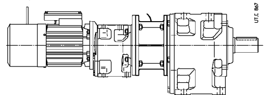
MLA montaggio nei gruppi (combinati) mounted onto combined units
